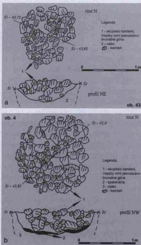
Ryc. 8. Malenin 153. Przykłady palenisk — plany ogółu i przekroje nr 4 (b), nr 43 (a), nr 77 (c). Rys. W. Dawidowicz
