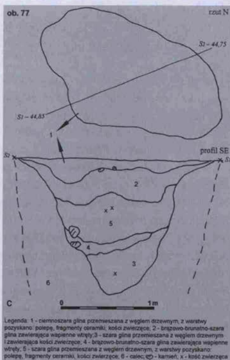
Ryc. 8. Malenin 153. Przykłady palenisk — plany ogółu i przekroje nr 4 (b), nr 43 (a), nr 77 (c). Rys. W. Dawidowicz
