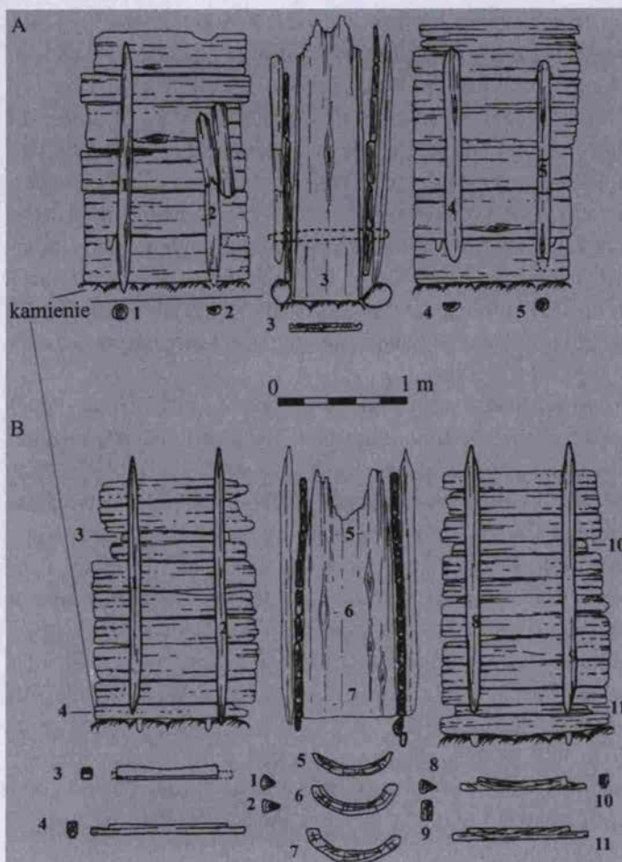
Ryc. 5. Rogaszyń, stan. 2-4, gm. Piątek, woj. łódzkie. Rozwinięcie ścian studni wczesnośredniowiecznych: A — obiekt nr 278; B — obiekt nr 280, wraz z przekrojami i rysunkami detali składowych
