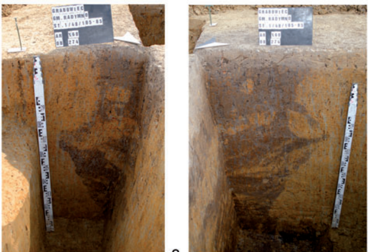
Ryc. 28. Grabowiec, stan. 1, gm. Radymno, woj. podkarpackie. Profile wybranych studni. (1) obiekt 159 (ar U61); (2) obiekt 274 (ar X68)
